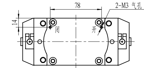
B底部通气款底部气孔尺寸示意
