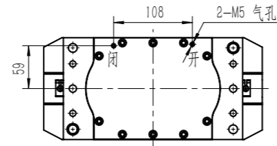
B底部通气款底部气孔尺寸示意
